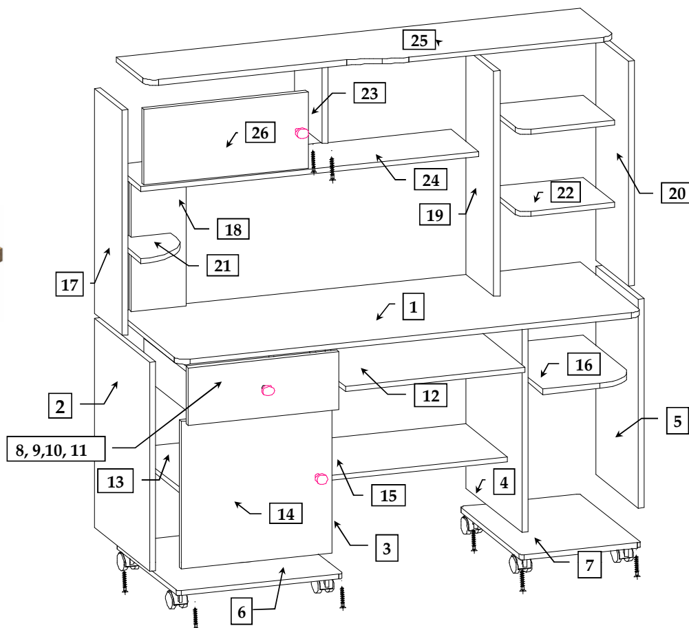
Комплектовочная ведомость на детали
