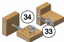
Эксцентриковая стяжка
